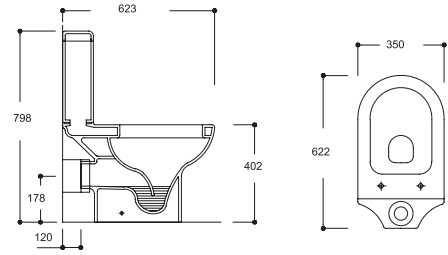
K003KLZ00 COMPACT KLOZET (ARKA ÇIKIŞLI) K001RZV REZERVUAR K004KLZ00 COMPACT CLOSET (P-TRAP) K001RZV CISTERN
